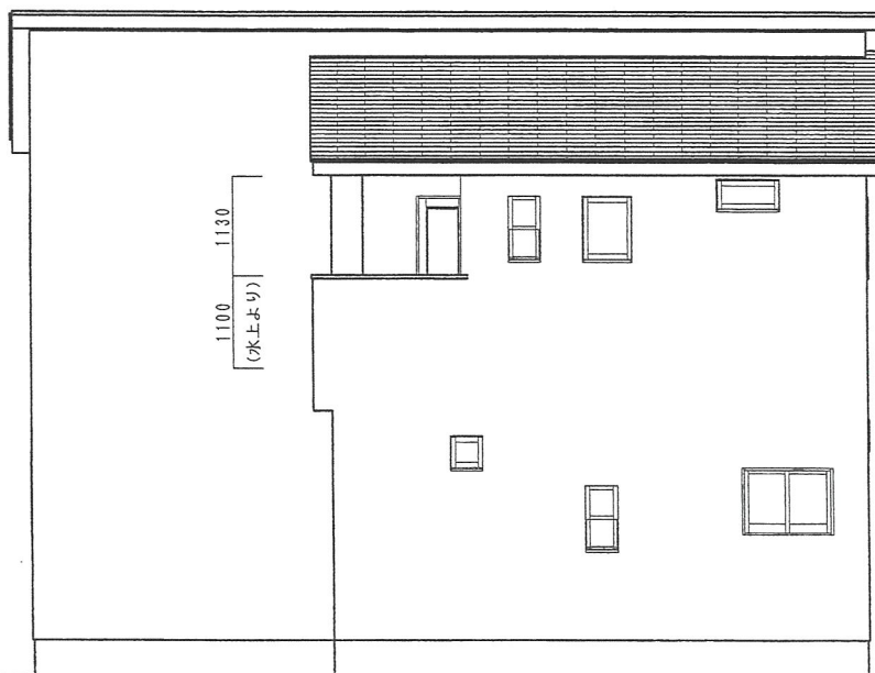
北側立面図
