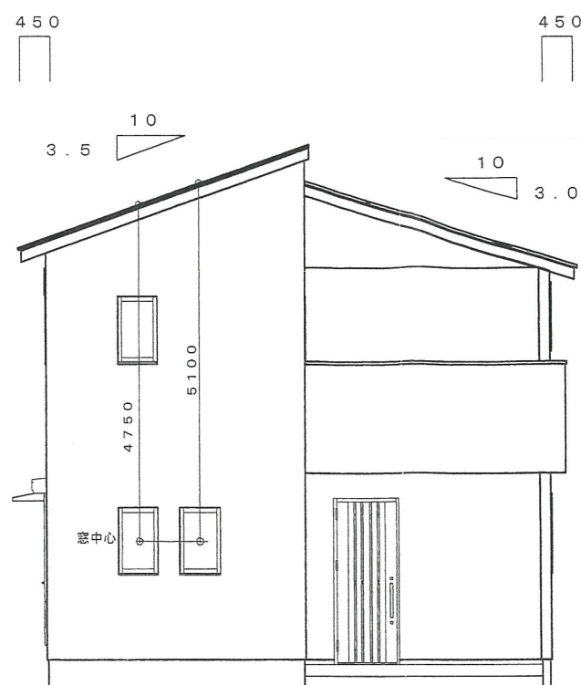
東側立面図
